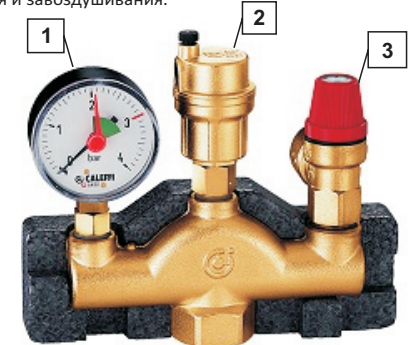
Рисунок 1. Группа безопасности котла: 1 - манометр, 2 - автоматический воздухоотводчик, 3 - предохранительный клапан
